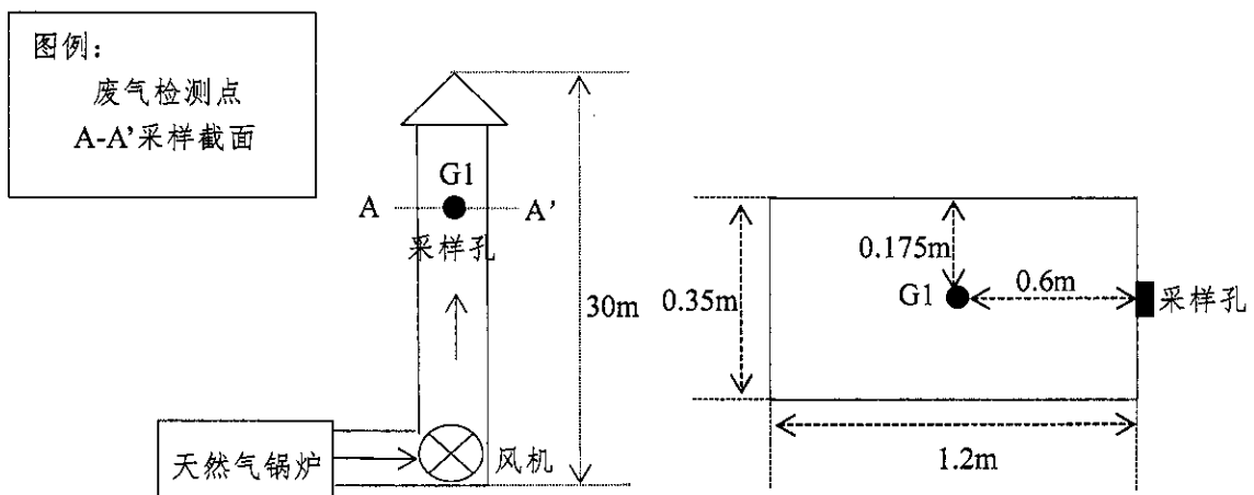
图二 有组织废气检测布点示意图
