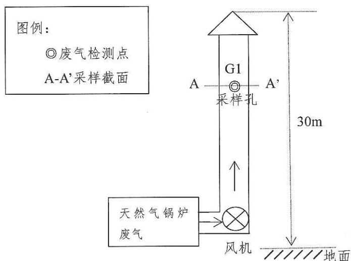
图二 有组织废气检测布点示意图
