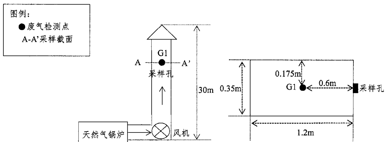
图三 有组织废气检测布点示意图
